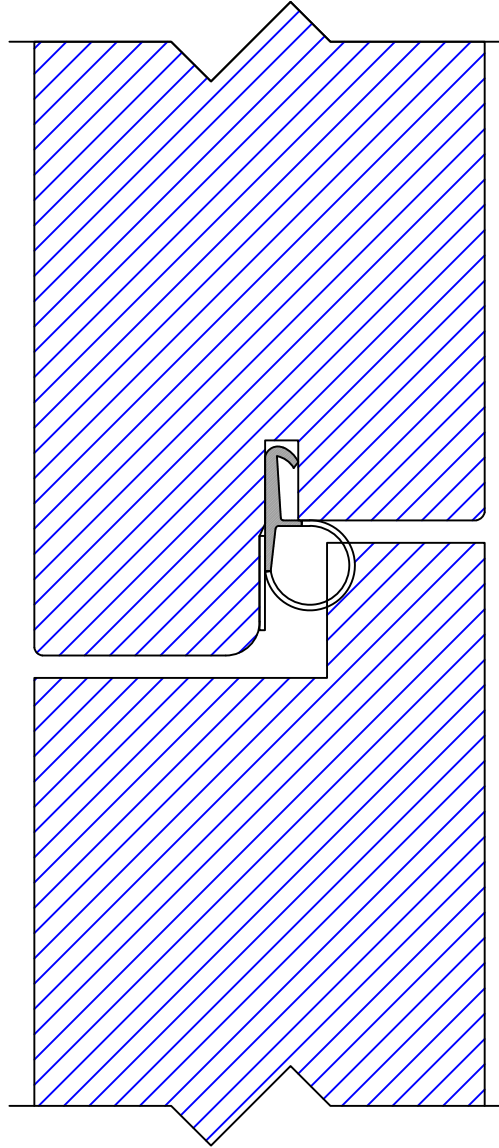
DEKO TD door top block
