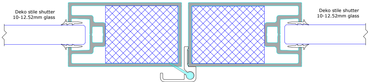
Double leaf door
