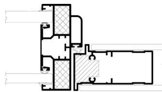
DEKO DG - Double glazed door
